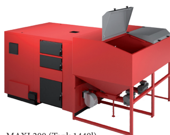
MAXI 200 (Tank 1440l)
